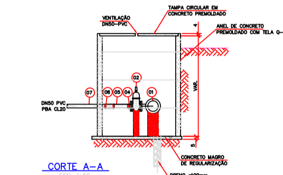
CORTE A-A
