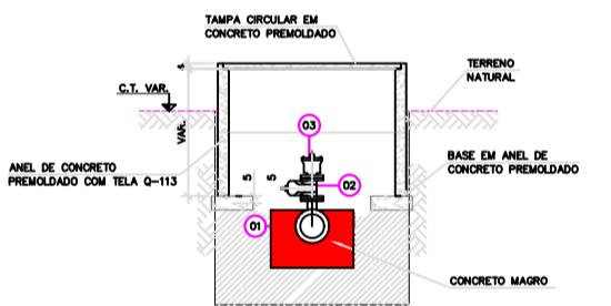
CORTE B-B
