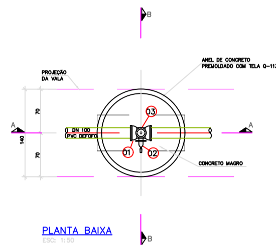
PLANTA BAIXA
